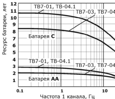
Рис. 1.1 – Ресурс батареи
