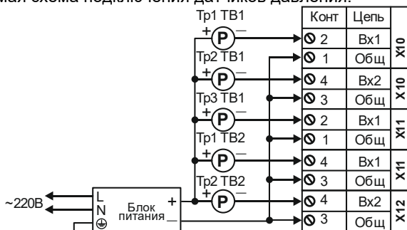
Рис. 4.4 – Пример подключения датчиков давления
