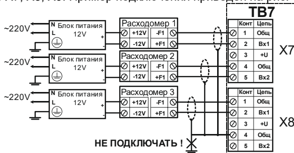
Рис. 4.2 Подключение импульсных линий связи
