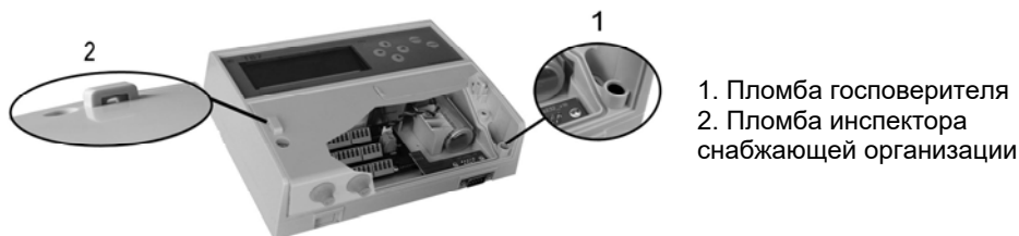
Рис. 1.2 – Места пломбирования вычислителя
