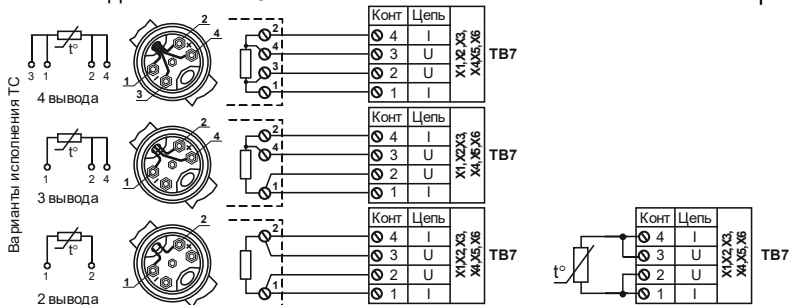
Рис. 4.3 - Варианты подключения ТС
