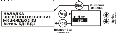
Рис. 3.12 – Сброс архива
