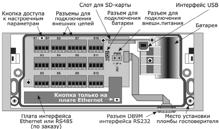
Рис. 2.2 – Вид на монтажный отсек при снятой крышке
